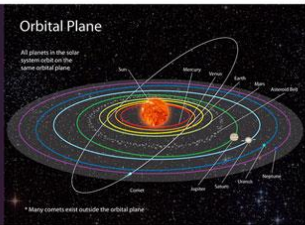
SYSTÈME SOLAIRE
